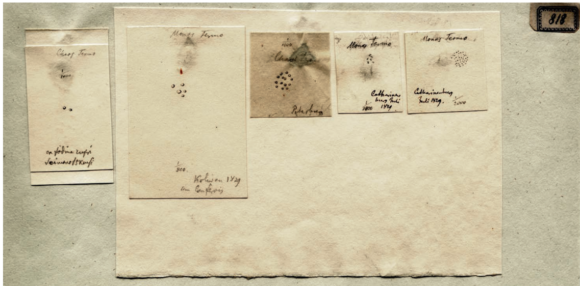
Abb. 4: Christian Gottfried Ehrenberg: Zeichnungen der Monas termo auf verschiedenen Stationen der russisch-sibirischen Reise: Soimonovskaja (Goldseife im mittleren Ural), Kolywan, St. Petersburg und Jekaterinburg. MfN, Mikropaläontologische Sammlungen, Ehrenberg-Sammlung, Zeichenblatt Nr. 818.
